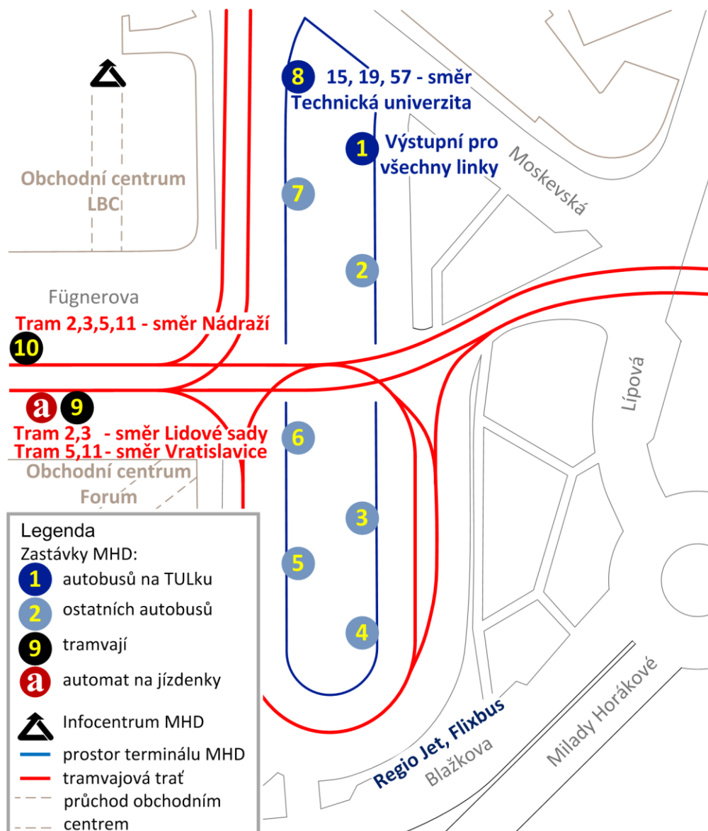
Obr. 17: Schéma rozmístění zastávek na terminálu MHD Fügnerova
